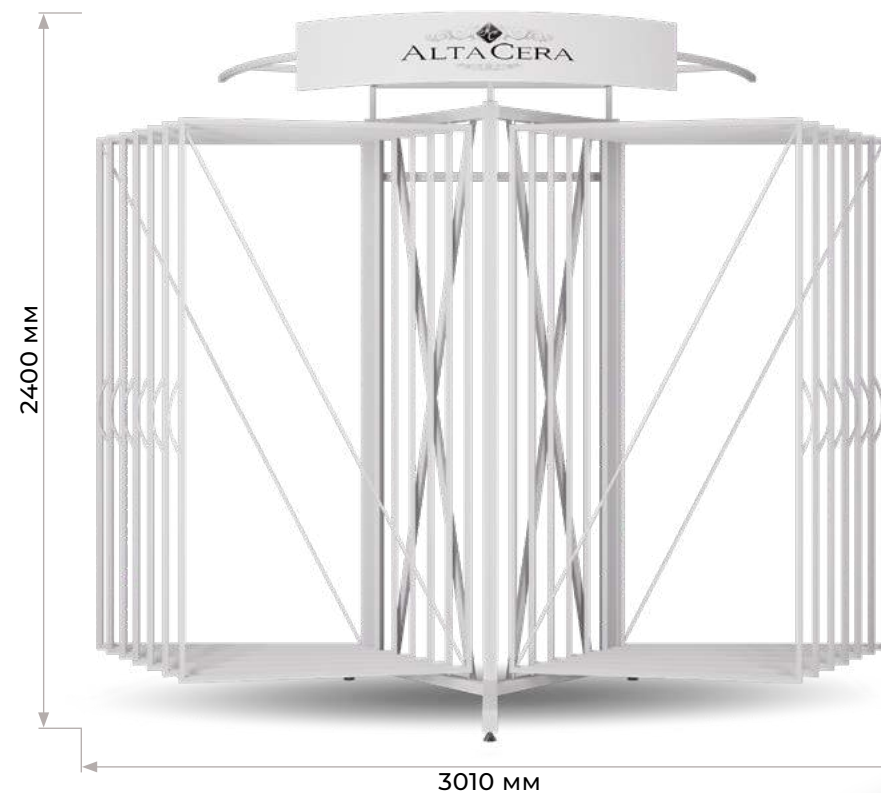
Размеры стенда для коллекционной плитки на 26 панелей 1000x1920 мм
